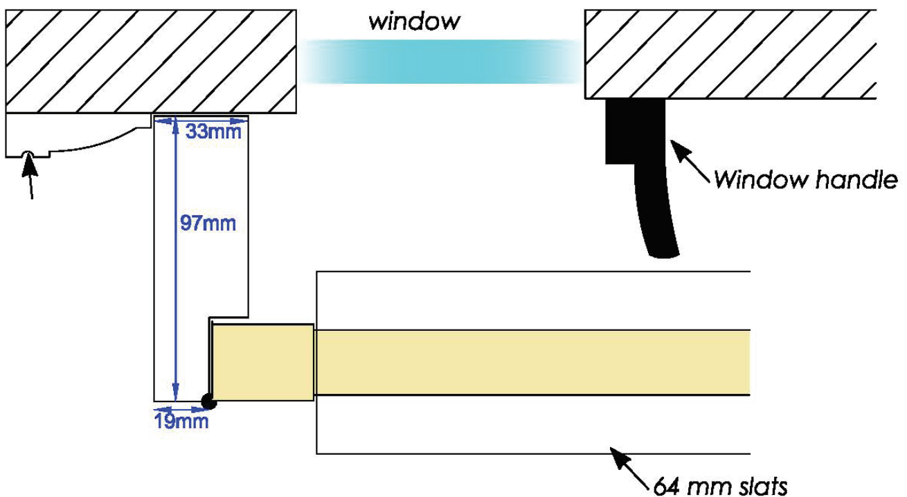
BOVENAANZICHT VAN RAAM & FRAME Getoond frame: 4038 Montage op de dag
